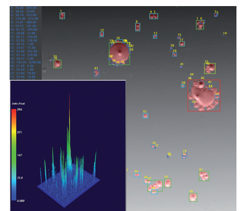
Abbildung 2: Inspektion beschichteter Metalloberflächen: Defekte unterschiedlicher Größen und Ausprägungen werden detektiert und bewertet.
